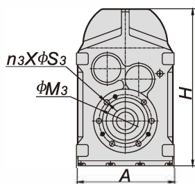
ショートフランジ取付
