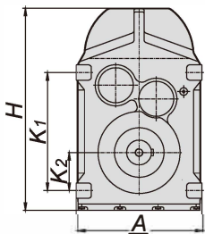
脚取付
