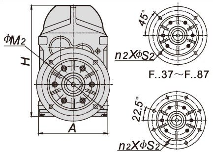
フランジ取付
