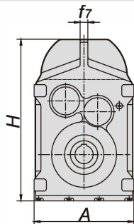
軸取付 (トルクアーム取り付けに適用)
